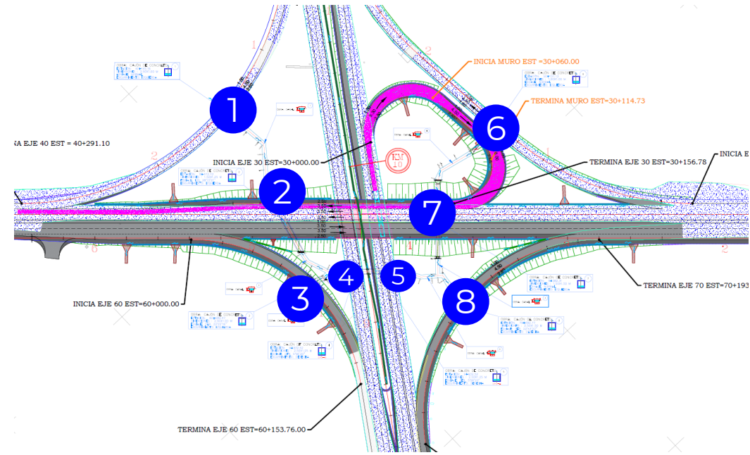
PLANTA CON UBICACIÓN DE OBRAS DE DRENAJE
