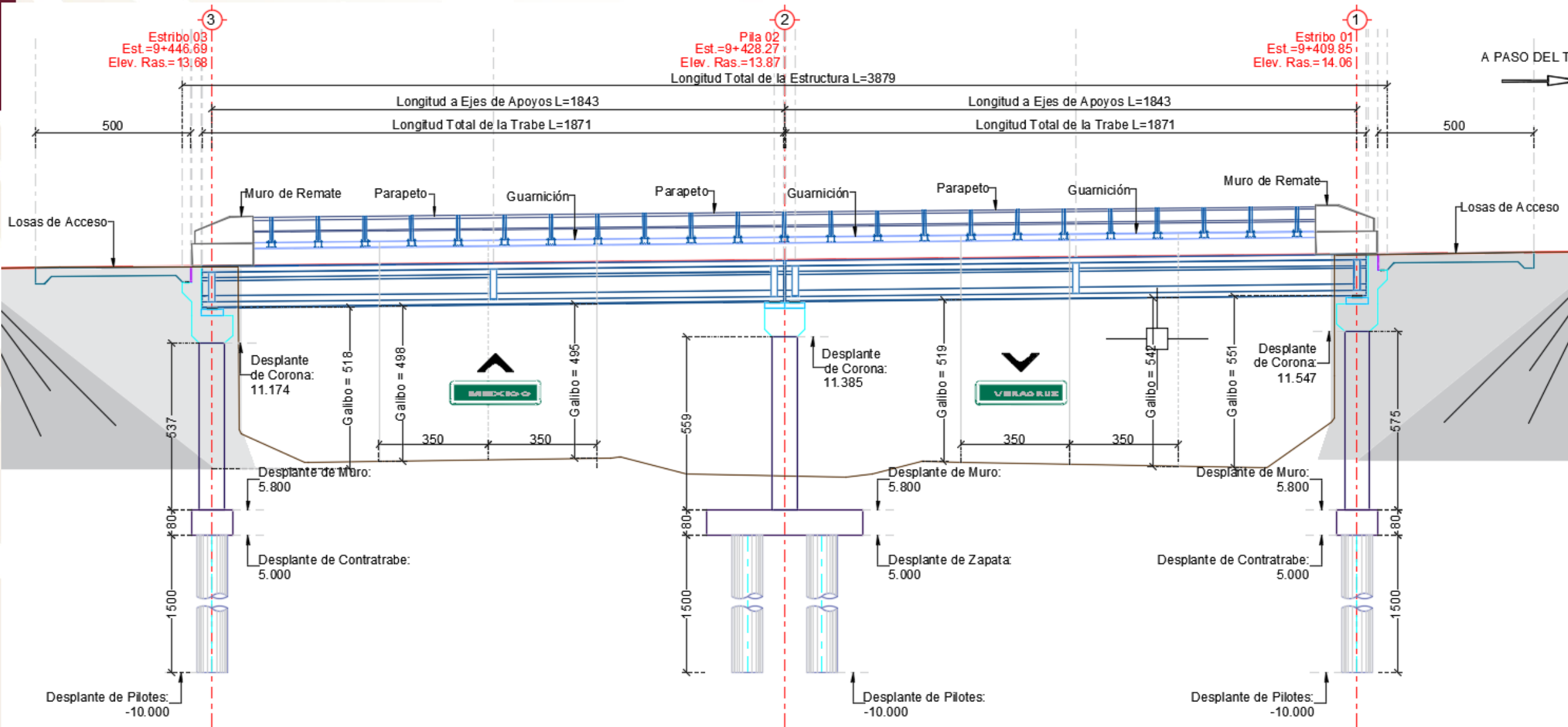
PERFIL ESTRUCTURAL
