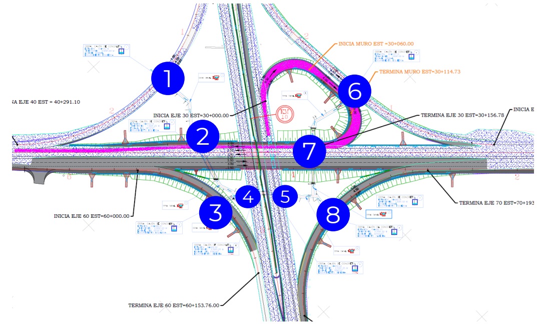
PLANTA CON UBICACIÓN DE OBRAS DE DRENAJE
