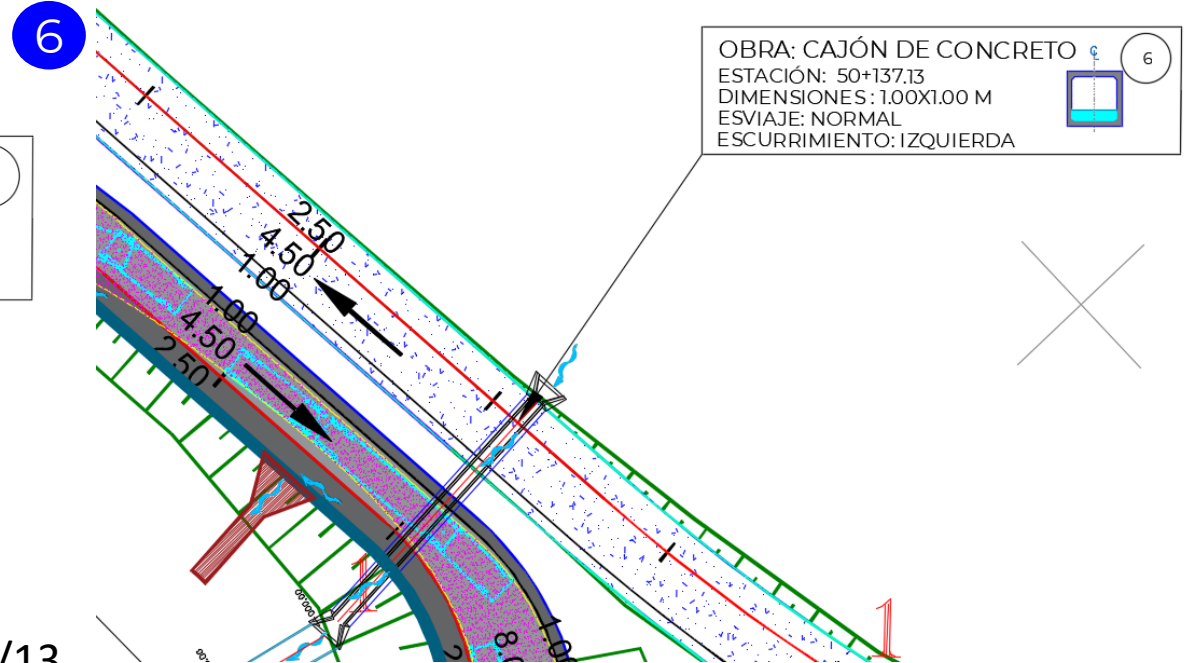
PLANTA CON UBICACIÓN DE OBRAS DE DRENAJE
